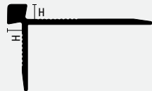
FVT 30 ASF
